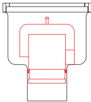
GVS Geruchsverschluss steckbar
