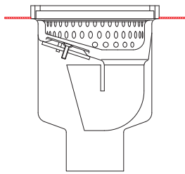
HF Haftflansch HFLALO Haftflansch mit Langloch
