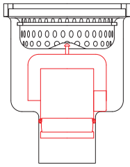
GVS Geruchsverschluss steckbar
