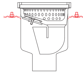
KMF Fest- und Losflansch mit Sickeröffnungen
