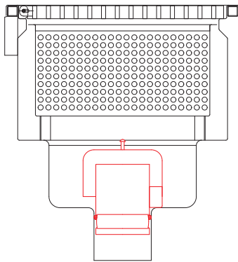
GVS Geruchsverschluss steckbar
