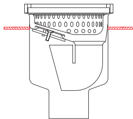
TGF Tragflansch
