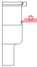
FDIN Fest- und Losflansch nach DIN 18534-2
