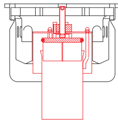
AS 14) Geruchsverschluss absperrbar
