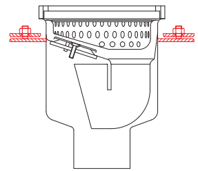
FDIN Fest- und Losflansch nach DIN 18534-2 mit Sickeröffnungen
