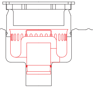
GVS Geruchsverschluss steckbar
