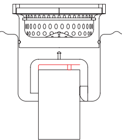
SBV Siebblech verschraubt SBS Siebblech gesteckt SBE Siebblech eingeschweißt
