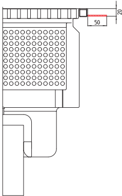
HF Haftflansch
