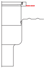
HF Haftflansch HFLALO Haftflansch mit Langloch
