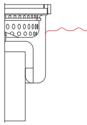
KBF Klebeflansch mit Sickeröffnungen
