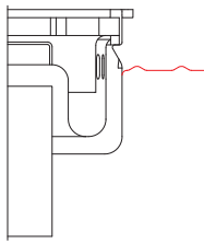
KBF Klebeflansch mit Sickeröffnungen
