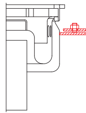
FDIN Fest- und Losflansch nach DIN 18534-2 mit Sickeröffnungen
