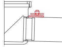
FDIN Fest- und Losflansch nach DIN 18534-2 mit Sickeröffnungen
