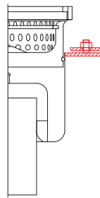
FDIN Fest- und Losflansch nach DIN 18534-2
