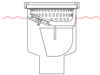
KBF Klebeflansch mit Sickeröffnungen
