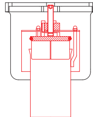
AS 14) Geruchsverschluss absperrbar
