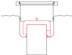
GV Glockengeruchsverschluss mit eingeschweißtem Standrohr
