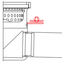
FDIN Fest- und Losflansch nach DIN 18534-2
