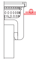
FDIN Fest- und Losflansch nach DIN 18534-2 mit Sickeröffnungen
